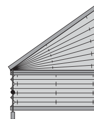
Typ 5a Snördrag Deko Plus
